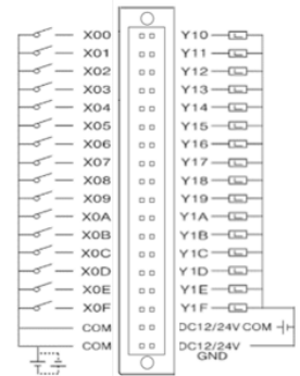
CM3-SP32PDCF 입력-출력
