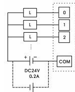
트랜지스터 출력
