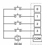
DC 입력
